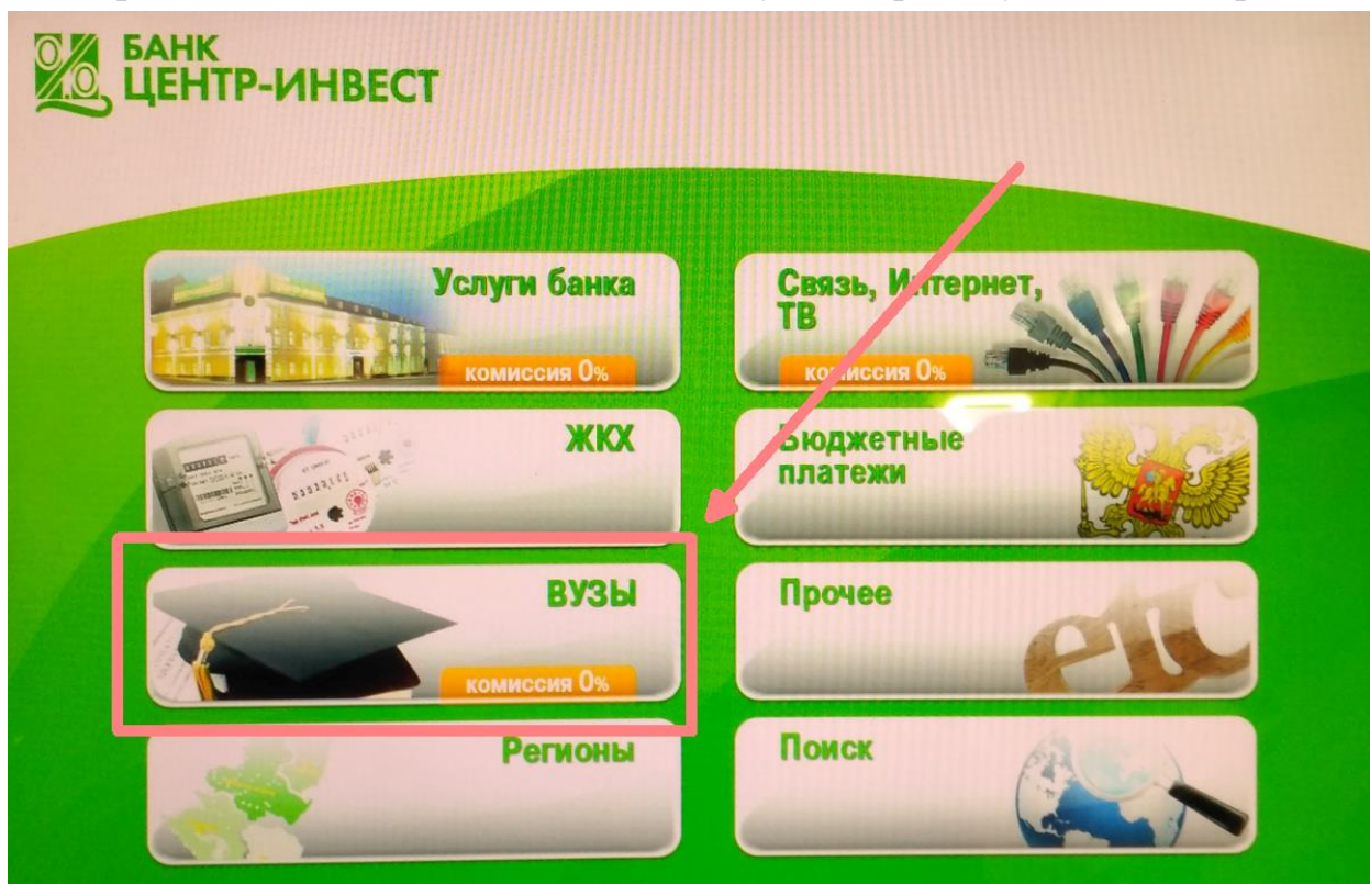
Рис. 1. Главное меню
